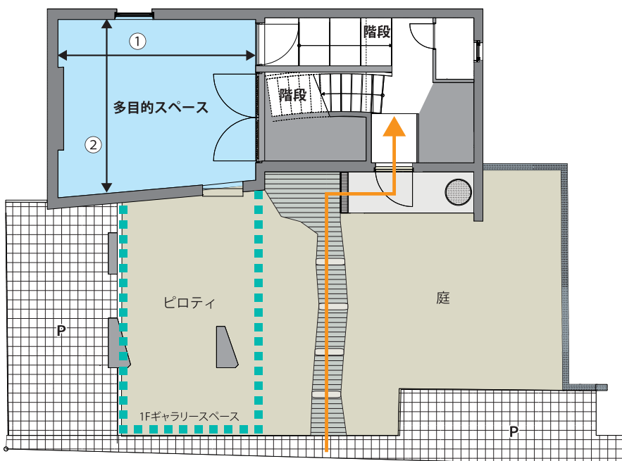
半地下平面図
